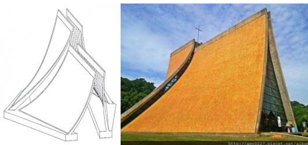
路思義教堂四片兩對雙曲拋物面圖及其建築成品
