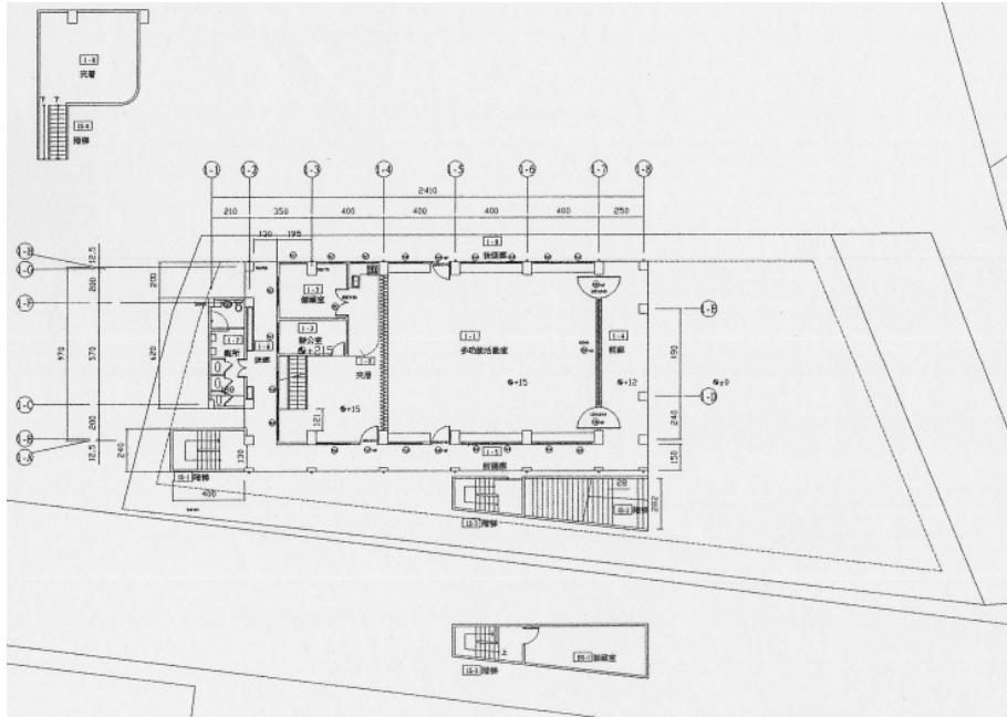
圖 26：守城活動中心 一樓平面圖
