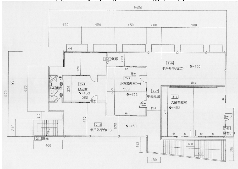
圖 27：守城活動中心 二樓平面圖
