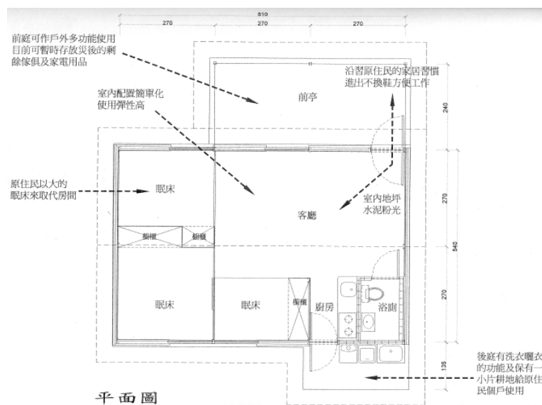
圖 4：邵族臨時家屋平面圖
