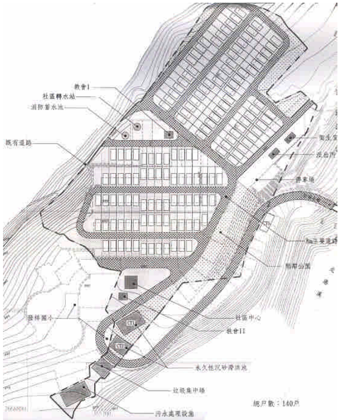
圖 14：瑞岩部落新址配置圖 12
