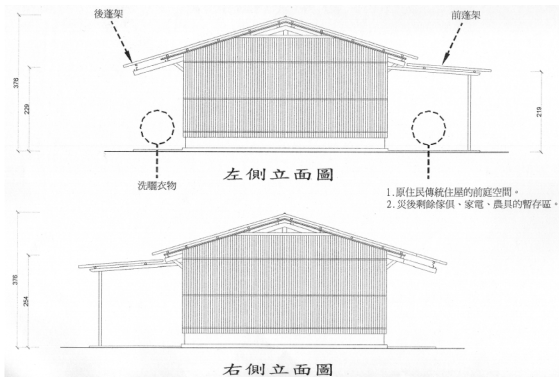
圖 5：邵族臨時家屋立面圖
