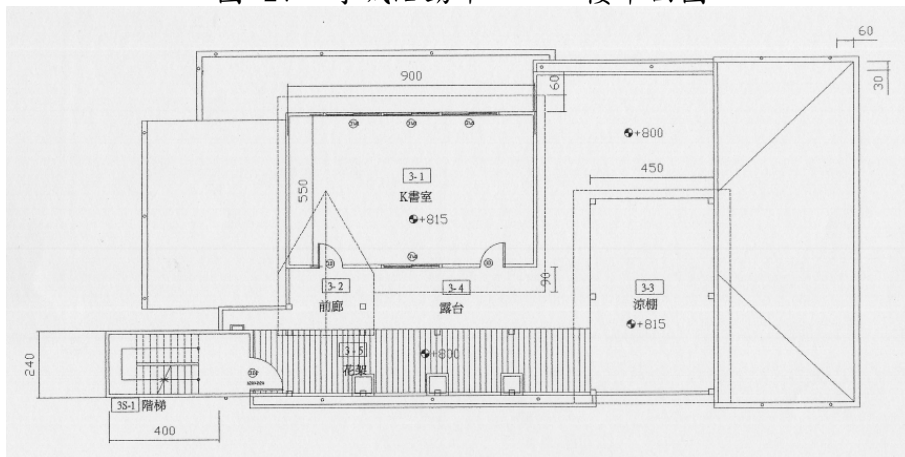
圖 28：守城活動中心 三樓平面圖
