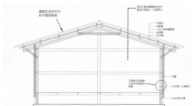
圖 6：邵族臨時家屋剖面圖
