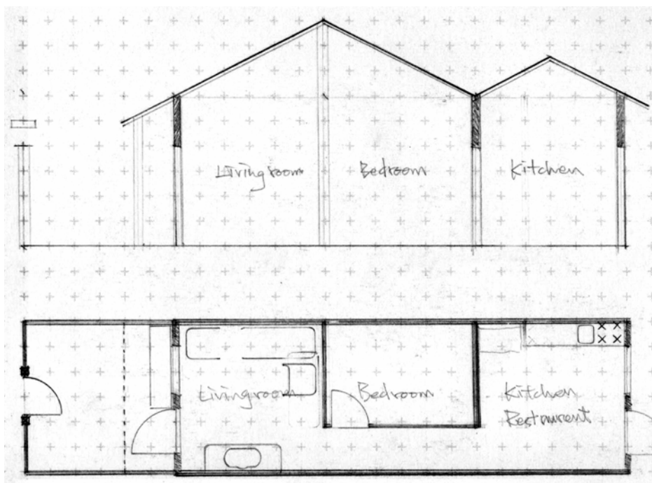
single-storied house / M.D.V. HISTORY HALL 一樓黑瓦厝 / 眷村歷史館
