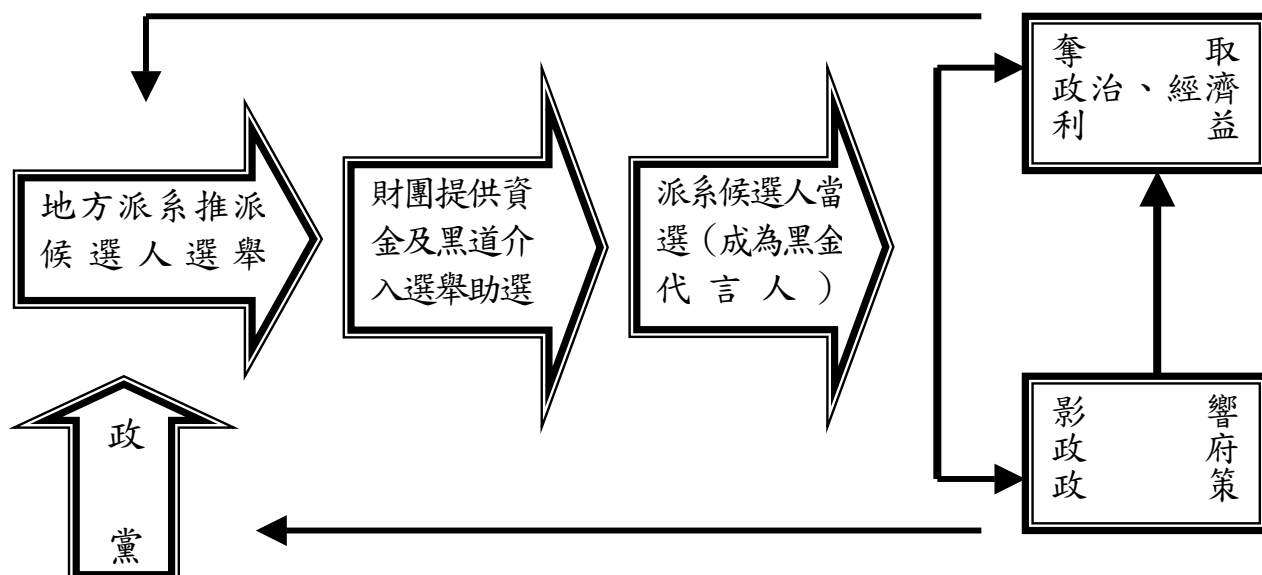
圖 1-1 研究架構
